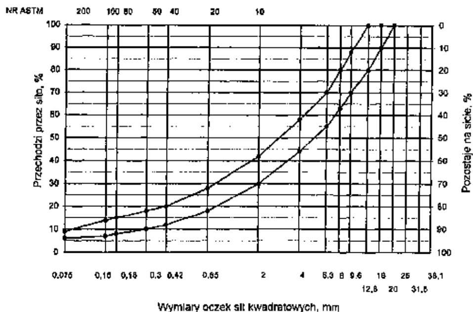
Rys. 6. Krzywe graniczne uziarnienia mieszanki mineralnej BA od 0 do 16 mm do warstwy ściernej nawierzchni drogi o obciążeniu ruchem od KR3 do KR6
