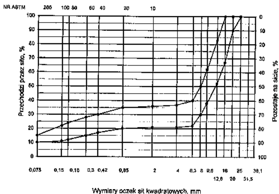
Rys. 5. Krzywe graniczne uziarnienia mieszanki mineralnej BA od 0 do 20 mm (mieszanka o nieciągłym uziarnieniu) do warstwy ściernej nawierzchni drogi o obciążeniu ruchem od KR3 do KR6
