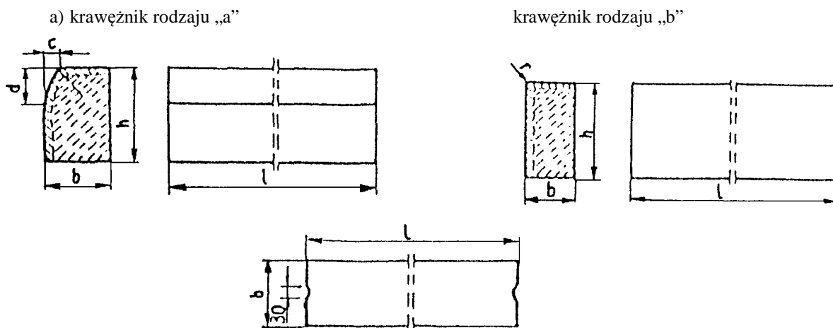
Rys. 1. Wymiarowanie krawężników
